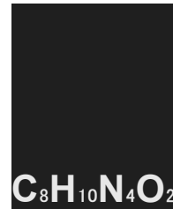
MOLÉCULA 4
