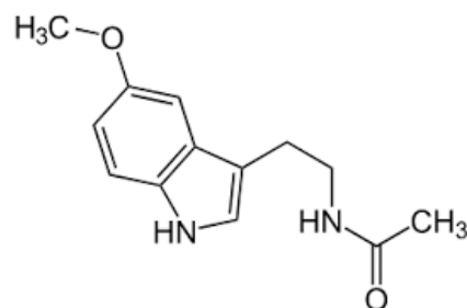
MOLÉCULA 10
