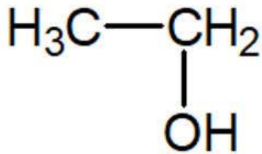
MOLÉCULA 9
