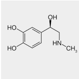
MOLÉCULA 1
